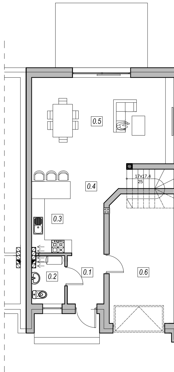
RZUT PARTERU
